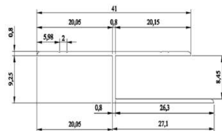
CODE : 2579 WEIGHT : 0,165 kg/m
