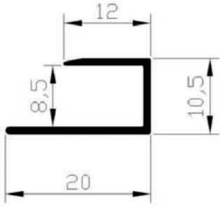
CODE : 110 WEIGHT : 0,104 kg/m
