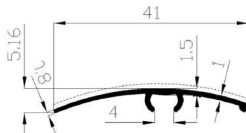
CODE : 510 WEIGHT : 0,128 kg/m
