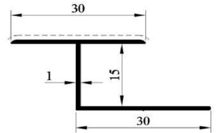
CODE : 412 WEIGHT : 0,201 kg/m
