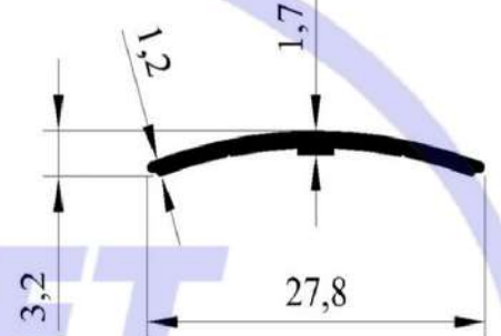
CODE : 313 WEIGHT : 0,093 kg/m
