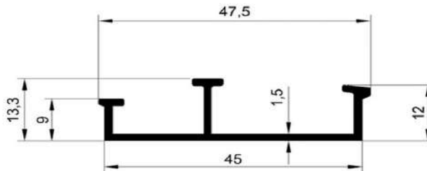
CODE : 4001 WEIGHT : 0,343 kg/m
