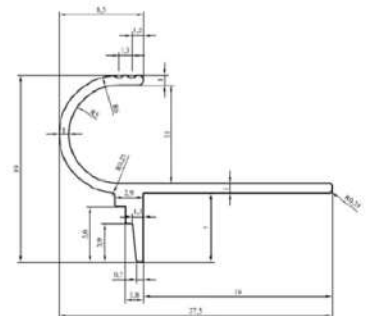
CODE : 2691 WEIGHT : 0,139 kg/m
