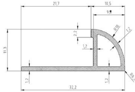
CODE : 2508 WEIGHT : 0,182 kg/m
