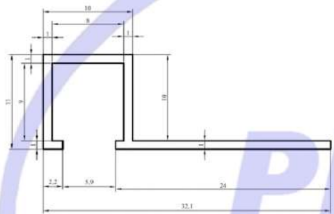
CODE : 2684 WEIGHT : 0,147 kg/m
