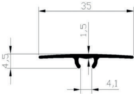
CODE : 212 WEIGHT : 0,126 kg/m
