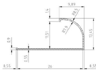
CODE : 2019-4 WEIGHT : 0,070 kg/m
