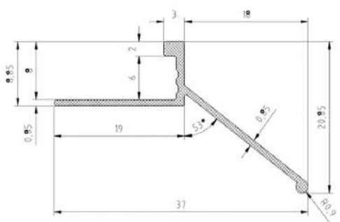
CODE : 2558 WEIGHT : 0,133 kg/m
