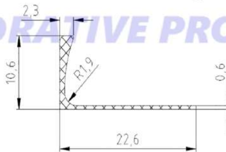
CODE : 2664 WEIGHT : 0,084 kg/m
