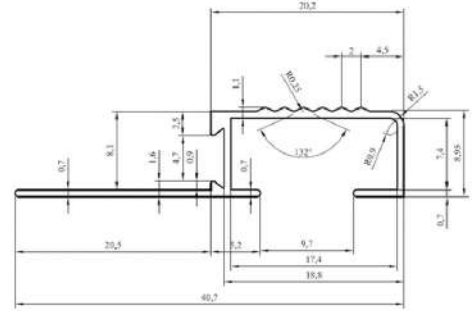
CODE : 2677 WEIGHT : 0,138 kg/m
