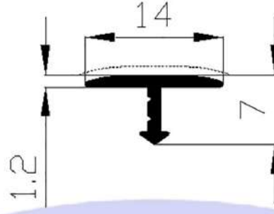
CODE : 215 WEIGHT : 0,065 kg/m
