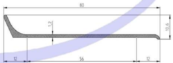
CODE : 8057 WEIGHT : 0,304 kg/m
