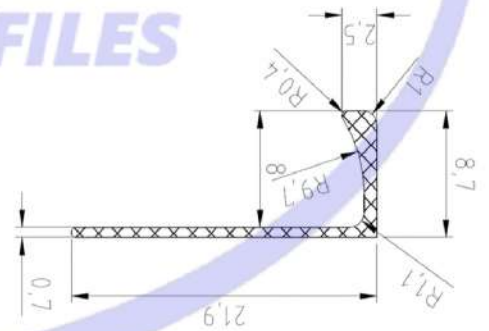
CODE : 2211-4 WEIGHT : 0,070 kg/m
