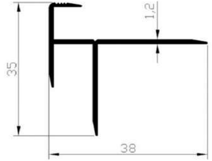
CODE : 612 WEIGHT : 0,224 kg/m
