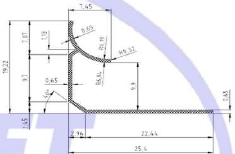
CODE : 2305 WEIGHT : 0,087 kg/m
