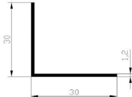
CODE : 30X30 WEIGHT : 0,191 kg/m
