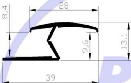
CODE : 413 WEIGHT : 0,205 kg/m
