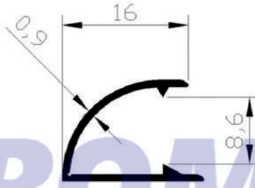
CODE : 114 WEIGHT : 0,103 kg/m
