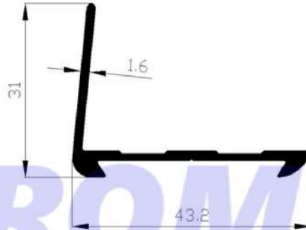
CODE : 614 WEIGHT : 0,360 kg/m
