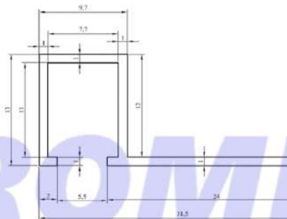
CODE : 2685 WEIGHT : 0,156 kg/m
