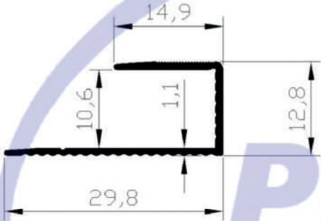
CODE : 113 WEIGHT : 0,144 kg/m
