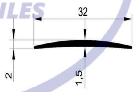
CODE : 211 WEIGHT : 0,103 kg/m
