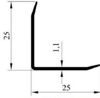
CODE : 816 WEIGHT : 0,138 kg/m
