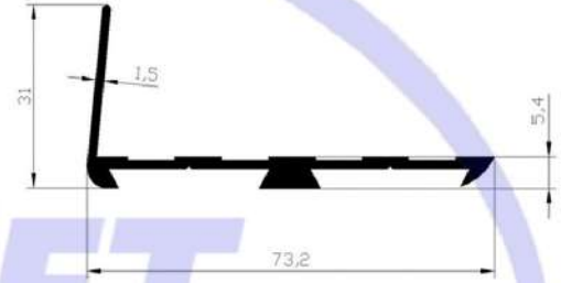
CODE : 615 WEIGHT : 0,587 kg/m
