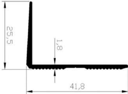
CODE : 617 WEIGHT : 0,302 kg/m
