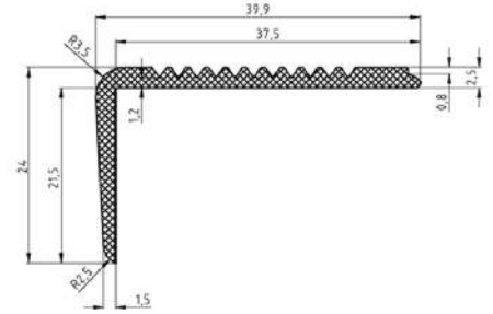
CODE : 2698 WEIGHT : 0,333 kg/m
