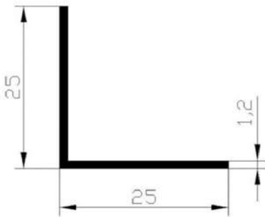
CODE : 25X25 WEIGHT : 0,159 kg/m
