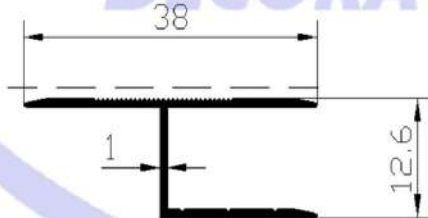
CODE : 417 WEIGHT : 0,171 kg/m
