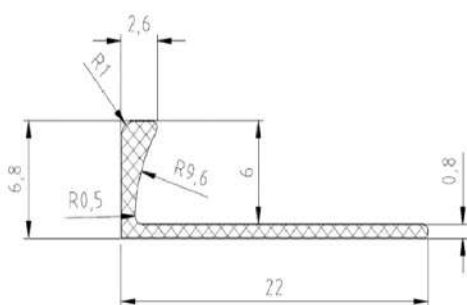
CODE : 2498 WEIGHT : 0,073 kg/m
