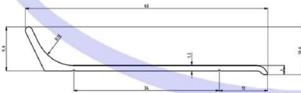
CODE : 3144 WEIGHT : 0,238 kg/m
