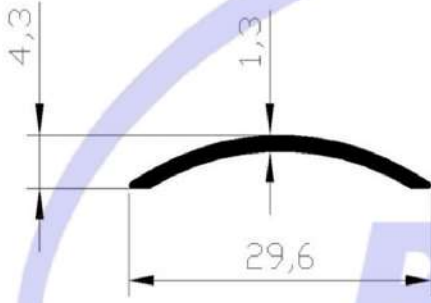
CODE : 311 WEIGHT : 0,103 kg/m
