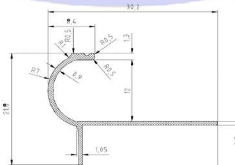
CODE : 2560 WEIGHT : 0,117 kg/m
