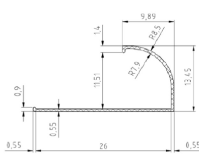
CODE : 2019-4 WEIGHT : 0,070 kg/m
