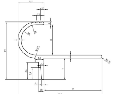
CODE : 2691 WEIGHT : 0,139 kg/m
