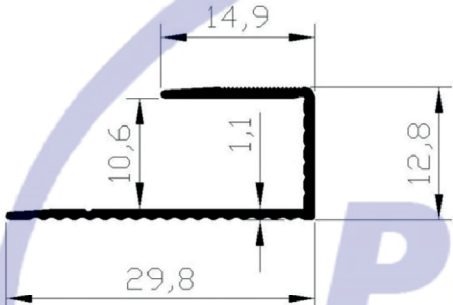
CODE : 113 WEIGHT : 0,144 kg/m
