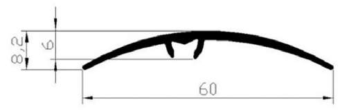
CODE : 519 WEIGHT : 0,295 kg/m
