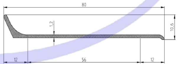
CODE : 8057 WEIGHT : 0,304 kg/m
