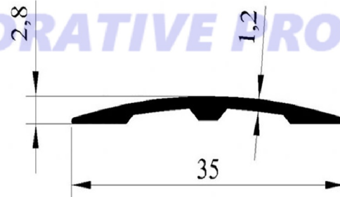
CODE : 312 WEIGHT : 0,146 kg/m
