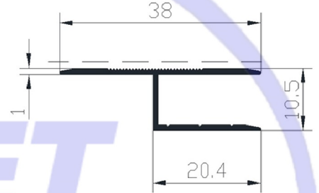
CODE : 416 WEIGHT : 0,165 kg/m
