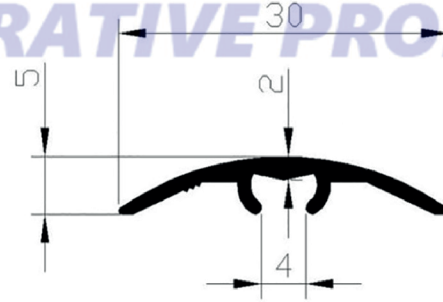
CODE : 210 WEIGHT : 0,140 kg/m
