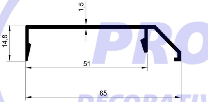
CODE : 4010 WEIGHT : 0,401 kg/m
