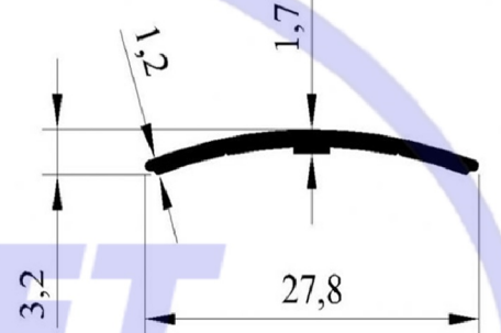
CODE : 313 WEIGHT : 0,093 kg/m
