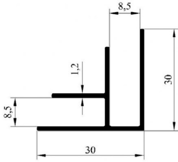
CODE : 627 WEIGHT : 0,317 kg/m
