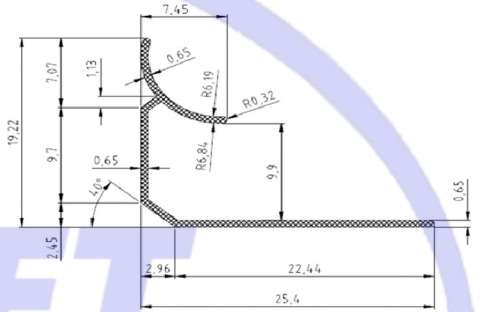
CODE : 2305 WEIGHT : 0,087 kg/m
