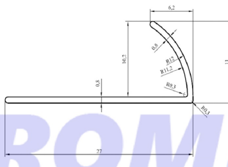
CODE : 2664 WEIGHT : 0,084 kg/m
