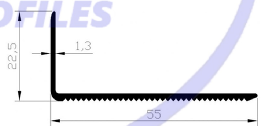
CODE : 615 WEIGHT : 0,587 kg/m
