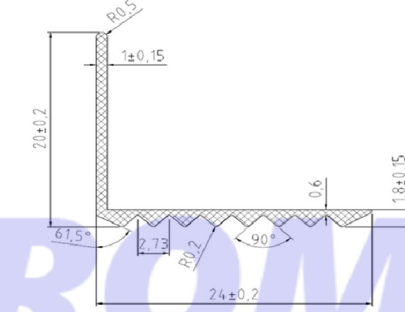
CODE : 8236 WEIGHT : 0,126 kg/m
