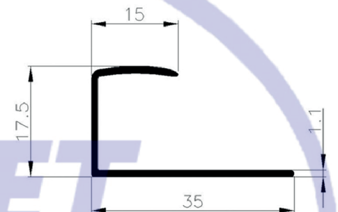
CODE : 119 WEIGHT : 0,190 kg/m
