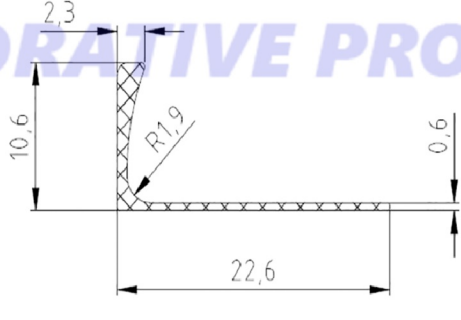
CODE : 2141 WEIGHT : 0,070 kg/m
