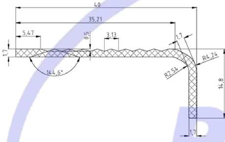
CODE : 1742 WEIGHT : 0,217 kg/m
