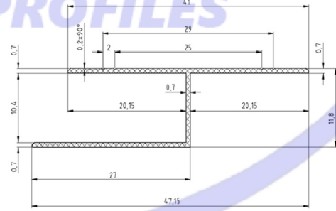
CODE : 2735 WEIGHT : 0,146 kg/m
