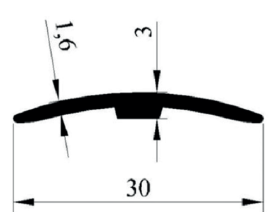
CODE : 310 WEIGHT : 0,147 kg/m
